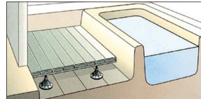
断面図
