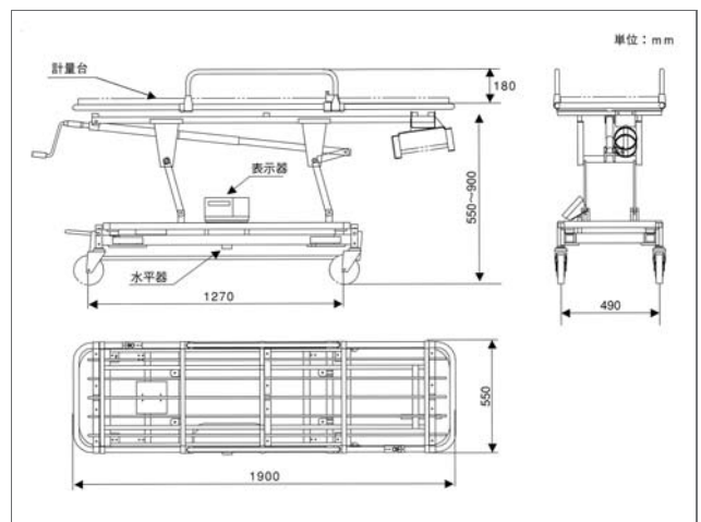
[寸法図]
