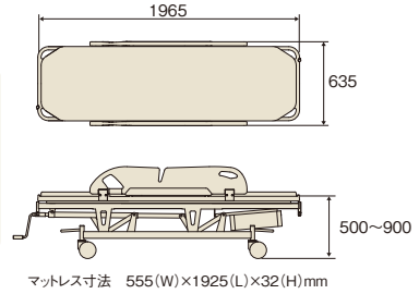
■寸法図(mm)
