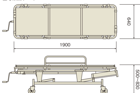
■寸法図(mm)
